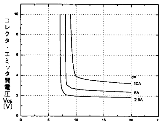
コレクタ・エミッタ間電圧-ゲート・エミッタ間電圧特性 ( T_j=125^\circ\text{C} ) <ブレーキ部> Collector-Emitter voltage vs. Gate-Emitter voltage <BRAKE>
