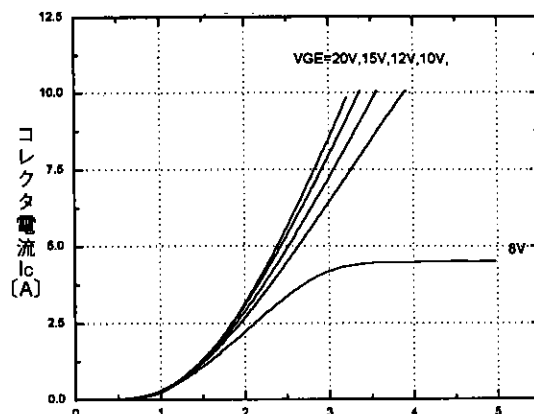
コレクタ電流-コレクタ・エミッタ間電圧特性 ( T_j=125^\circ\text{C} ) <ブレーキ部> Collector current vs. Collector-Emitter voltage <BRAKE>
