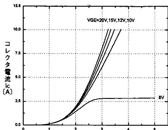
コレクタ電流-コレクタ・エミッタ間電圧特性 ( T_j=25^\circ\text{C} ) <ブレーキ部> Collector current vs. Collector-Emitter voltage <BRAKE>
