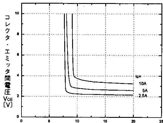
コレクタ・エミッタ間電圧-ゲート・エミッタ間電圧特性 ( T_j=25^\circ\text{C} ) <ブレーキ部> Collector-Emitter voltage vs. Gate-Emitter voltage <BRAKE>
