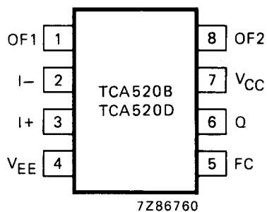
Fig. 2 Pinning diagram.
